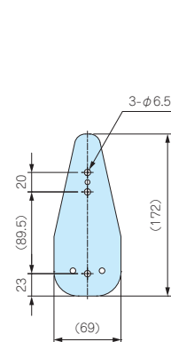
壁付ブラケット寸法
